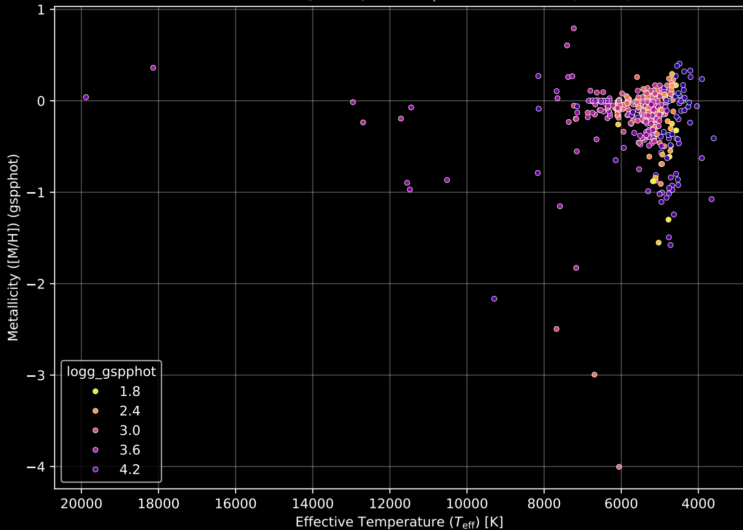
APOGEE DR17 Field: [180-04] Stellar Population Parameters (n= 418)
